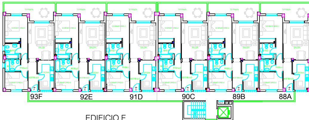
EDIFICIO F PLANTA COTA +103.40
