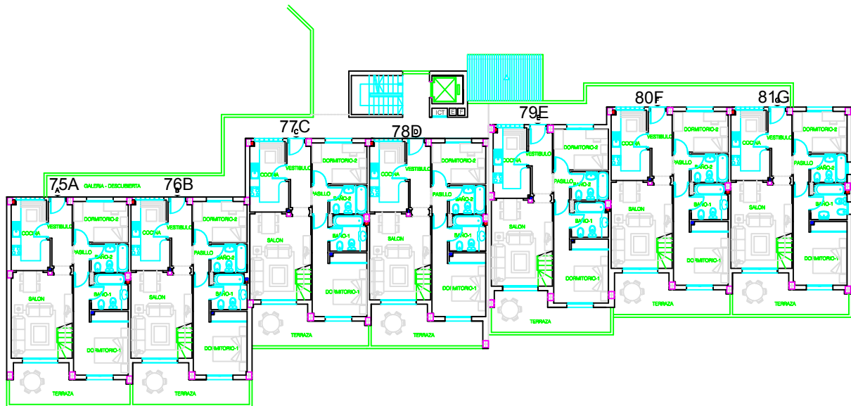
EDIFICIO E PLANTA COTA +100.60
