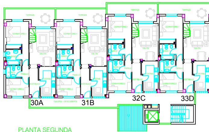
PLANTA SEGUNDA COTA +106,20
