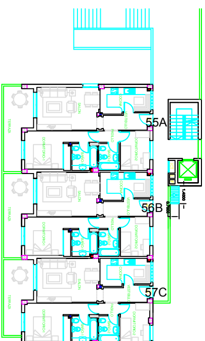
EDIFICIO D COTA +98,20
